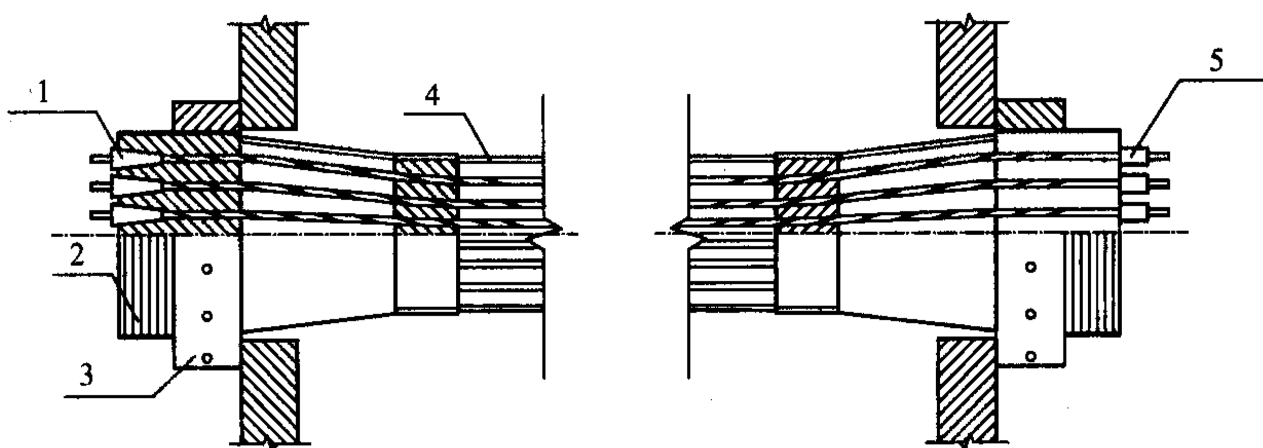
图 5.8.1-1 钢绞线拉索
