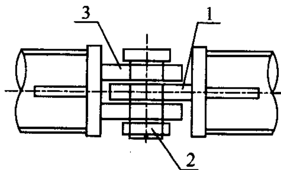
图 5.6.1 销轴式节点
