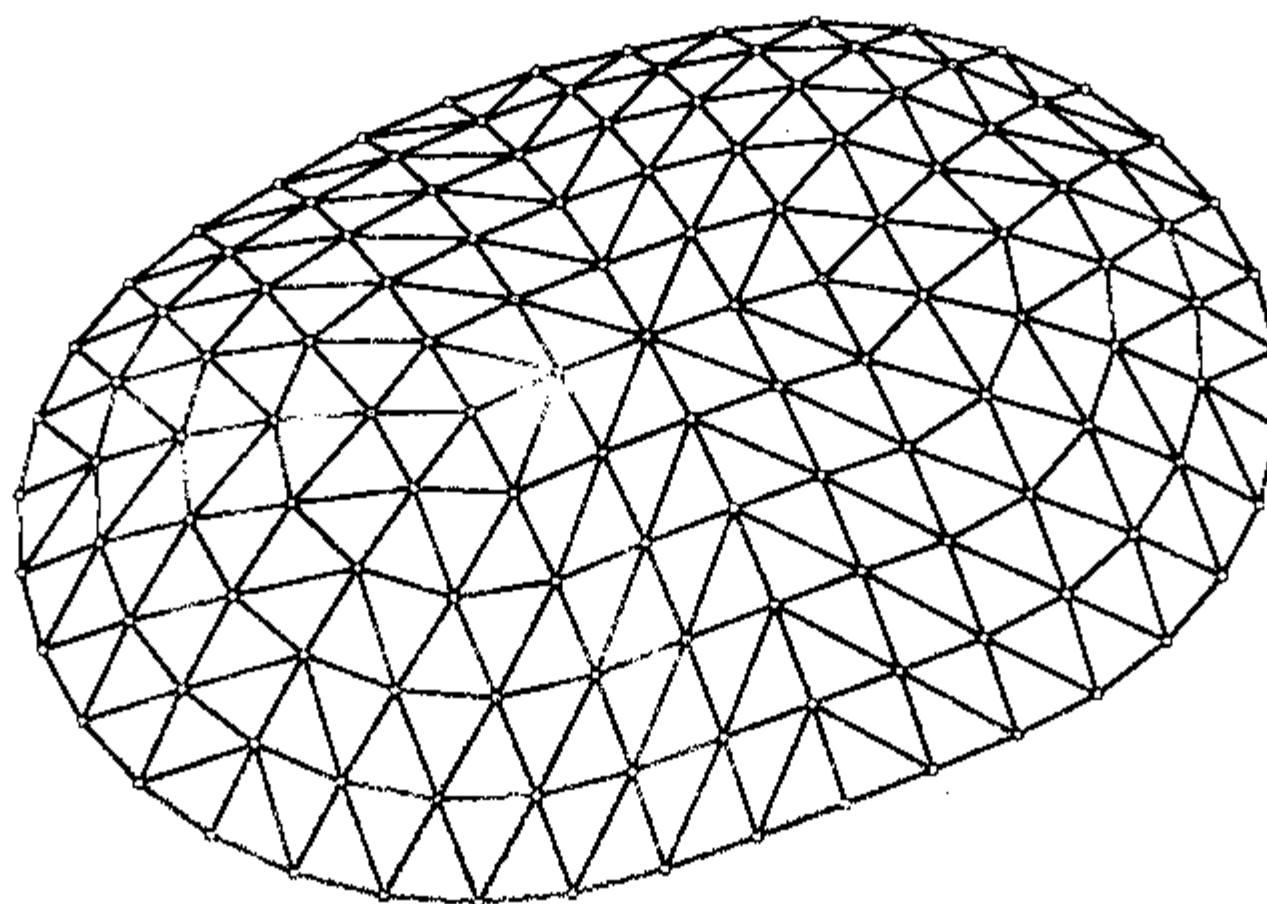
(c) 椭圆底面网格
