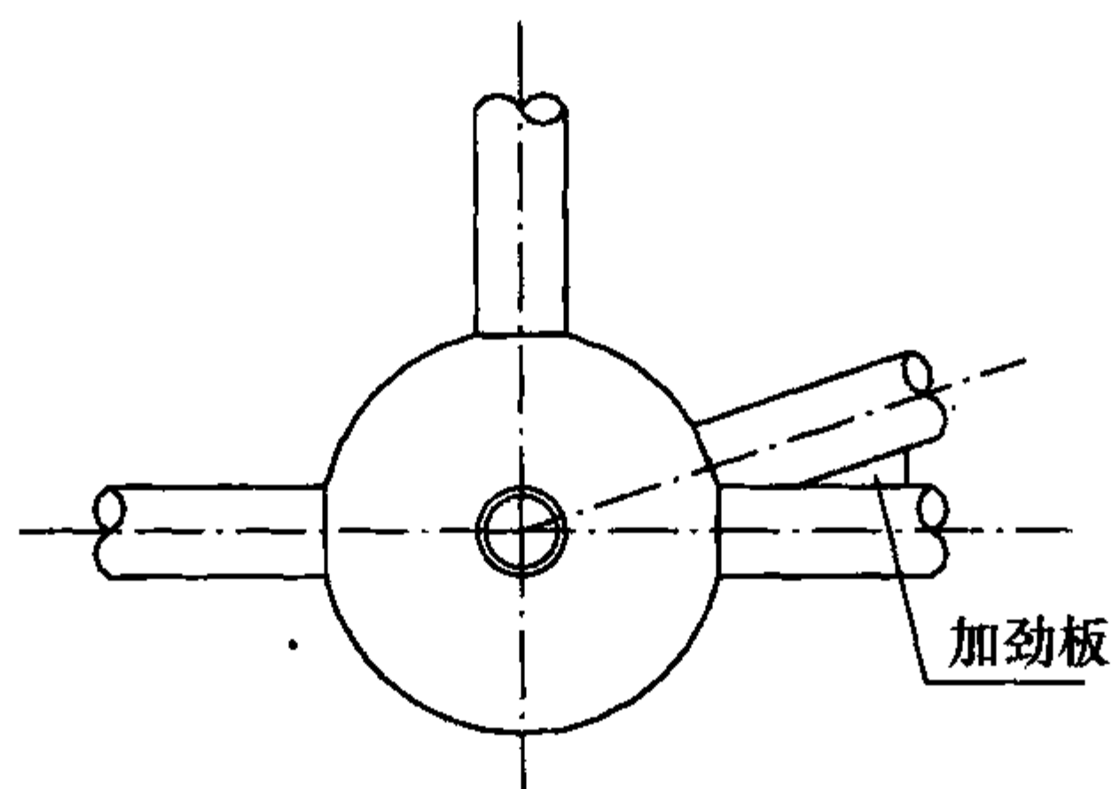
图 5.2.7-1 汇交杆件连接
